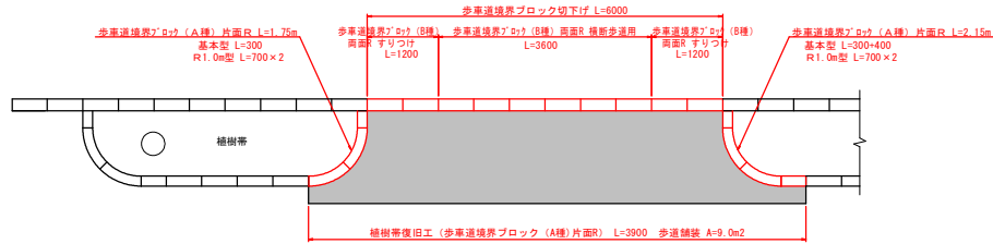
平面图 S=1/50
