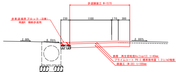
歩道切下げ図 S=1:20
