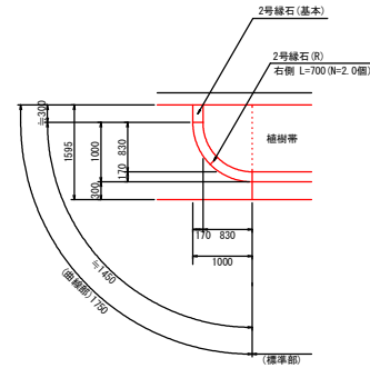
曲線部詳細図 S=1:50
