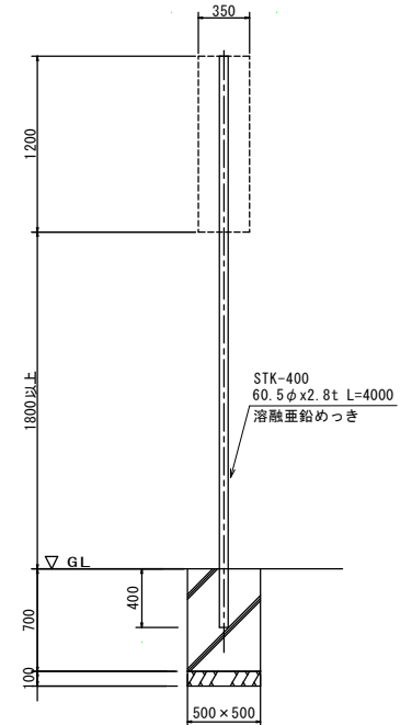
標識構造図 SC=1:20
