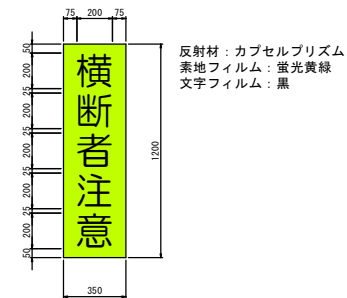
標識レイアウト SC=1:15
